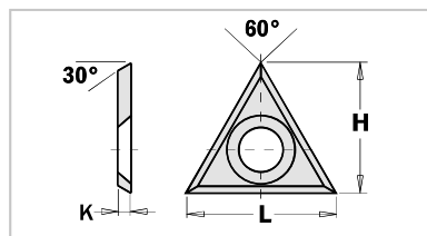
Płytki wymienne do fazowania i frezowania
